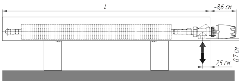
Вид для исполнения "нв" (нерегулируемая высота)
