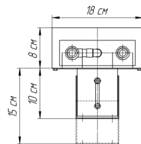
Исполнение "рв" (регулируемая высота)
