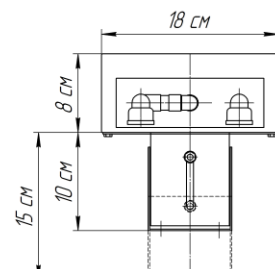
Исполнение "рв" (регулируемая высота)
