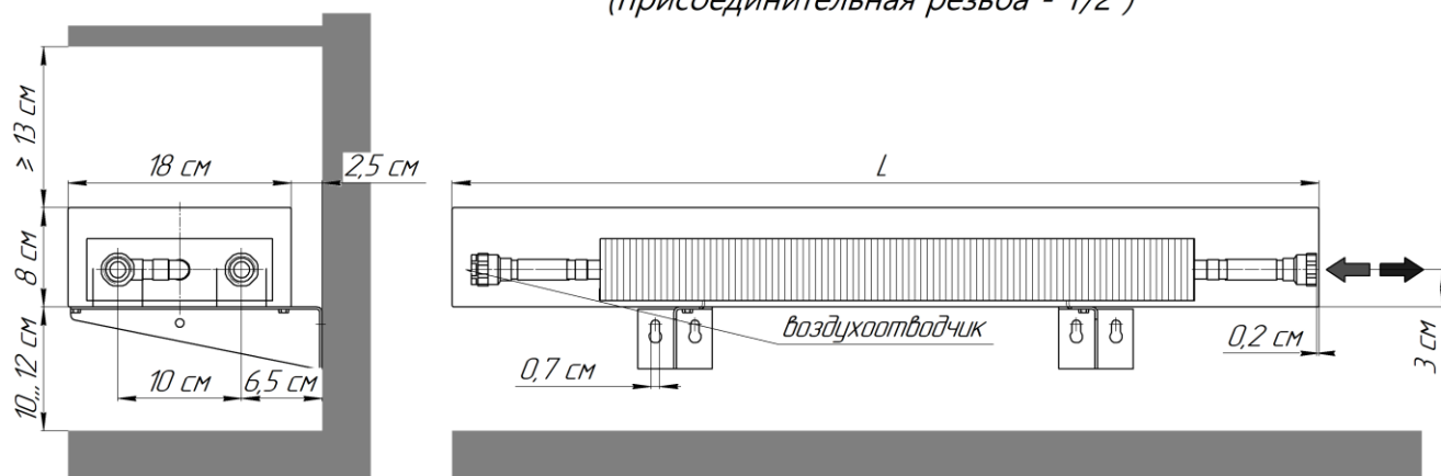
Настенный конвектор "Элегант - мини 180x80-1,5то бок Стен прав" с правосторонним боковым присоединением (левосторонне - зеркально) (присоединительная резьба - 1/2")
