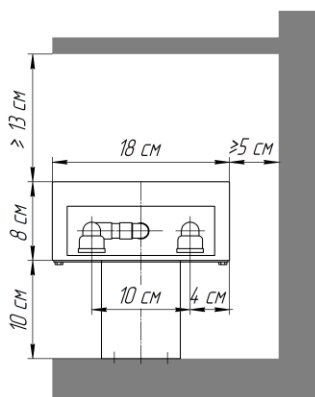
Исполнение "нв" (нерегулируемая высота)
